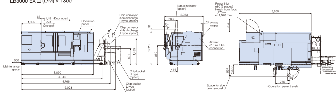
LB3000 EX III (L/M) × 1300
