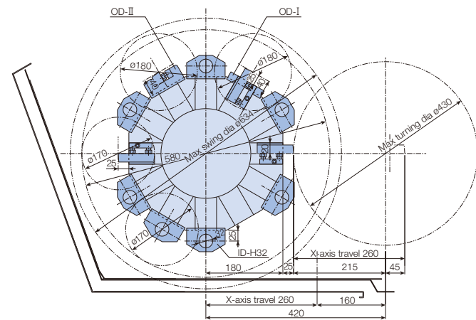
LB2000 EX III (L)
