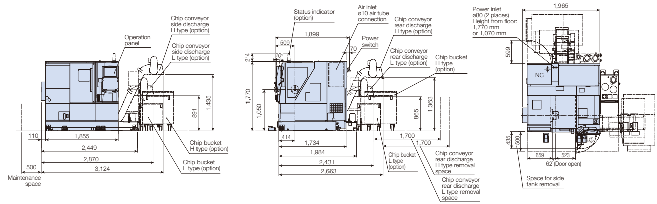
LB3000 EX III (L/M) × 500
